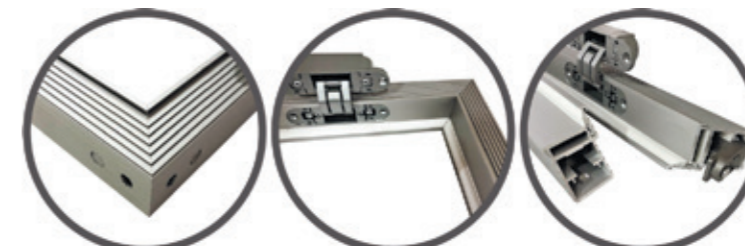
АЛЮМІНІЄВА ДВЕРНА КОРОБКА ПРИХОВАНОГО МОНТАЖУ / ALUMINUM DOOR BOX OF HIDDEN INSTALLATION Універсальна, для внутрішнього та зовнішнього відкриття / Universal, for internal and external opening
