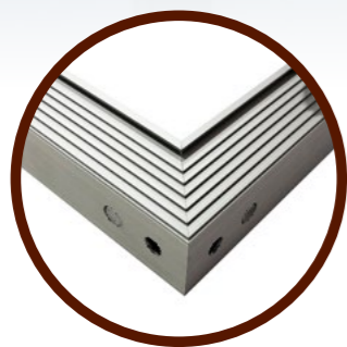
АЛЮМІНІЄВА ДВЕРНА КОРОБКА ПРИХОВАНОГО МОНТАЖУ / THE ALUMINIUM DOOR BOX OF HIDDEN INSTALLATION Універсальна, для внутрішнього та зовнішнього відкриття / Universal, for internal and external opening
